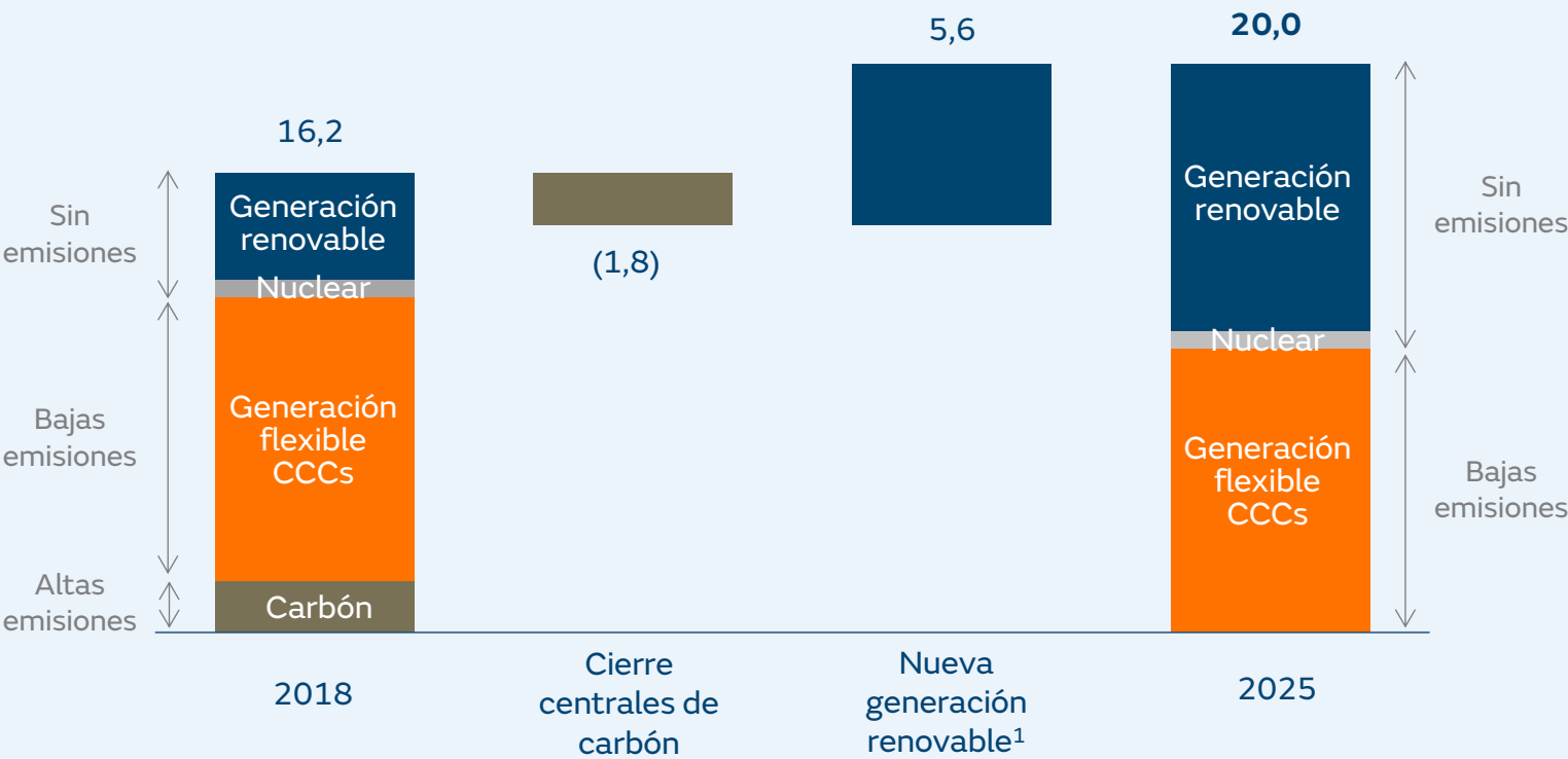
Capacidad de generación en operación (GW)
